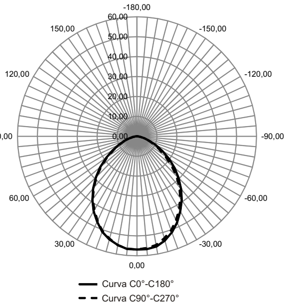
Distribución Intensidad Luminosa [cd]
